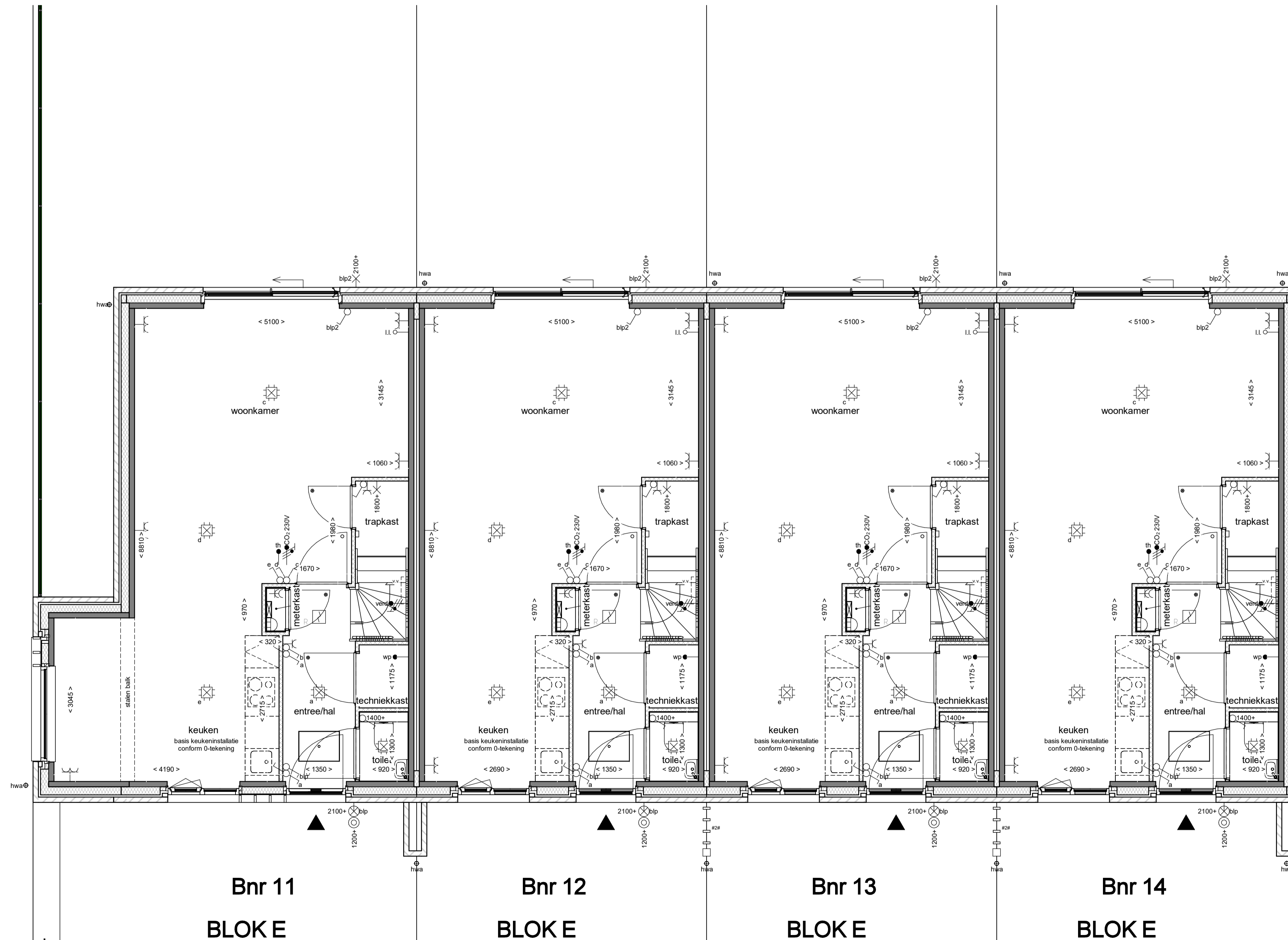
begane grond
